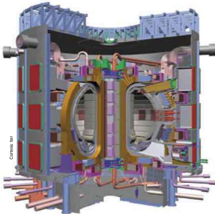
Vista em corte do dispositivo de fusão Iter. O dispositivo se baseia no conceito do tokamak, no qual gás quente é confinado em um toro, ou vaso em forma de donut, com o uso de um campo magnético. O gás será aquecido a mais de 100 milhões de graus Celsius e produzirá 500 megawatts de energia de fusão. A pessoa na parte inferior da imagem dá uma idéia do tamanho do dispositivo
